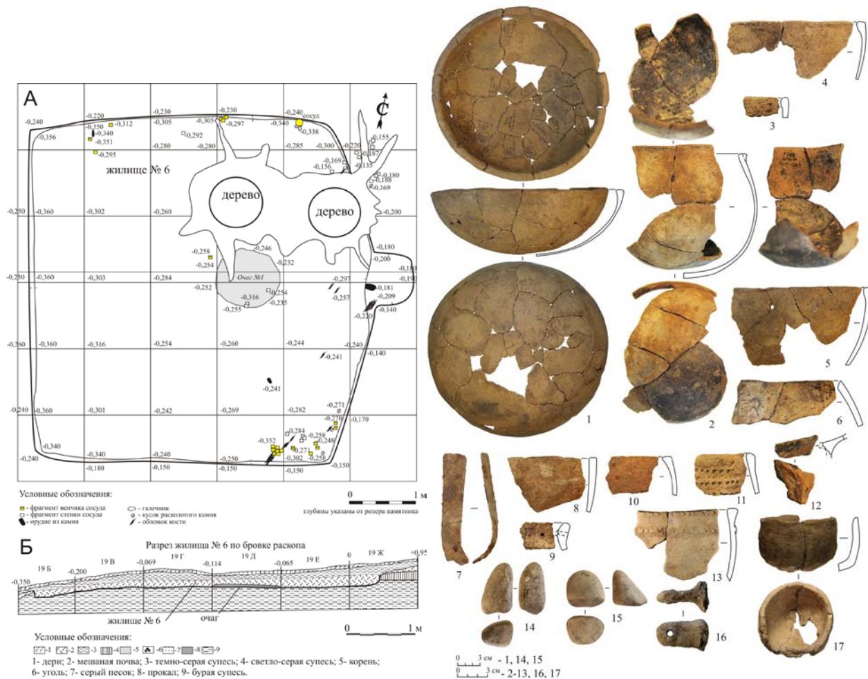
Рис. 1. План (А) и разрез (Б) жилища № 6 поселения Дом Отдыха-3.
